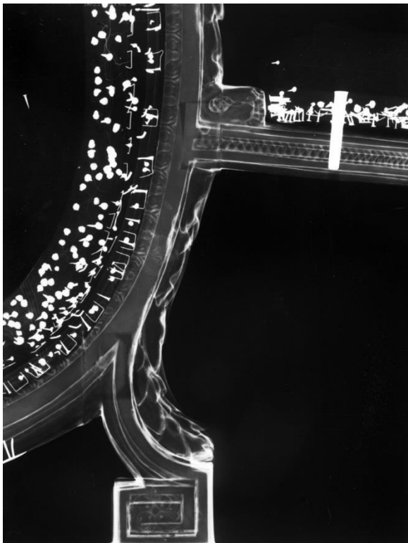
Fotel, nr inw. 146/4, fotografie RTG
